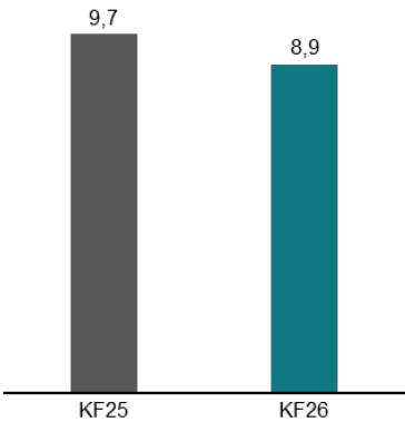
Figur 1.4 Udvikling i reduktionsmankoen til 100 pct. mål i 2050 i KF25 og KF26, mio. ton CO 2 e
